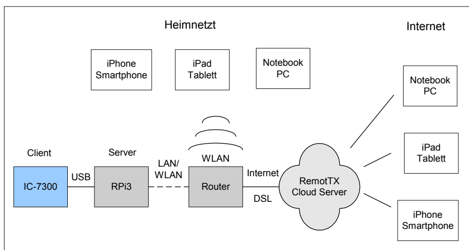
Bild 2: IC-7300 mit RPi3 ins Internet
