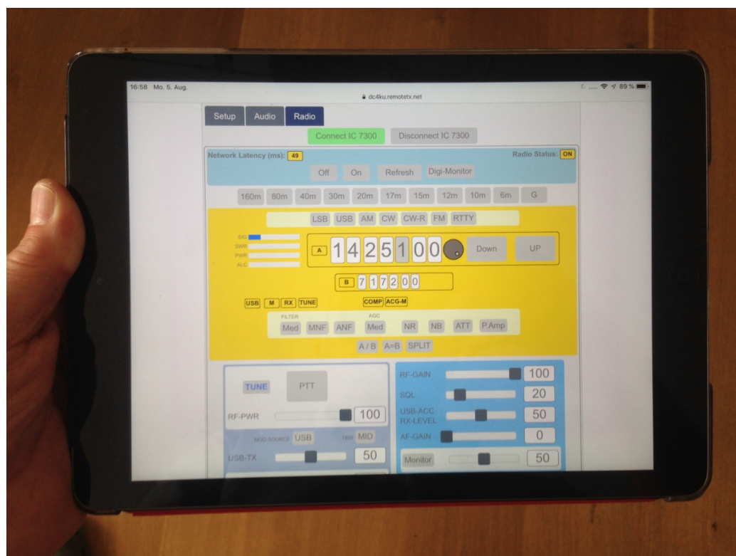
Bild 1: Fernsteuerung des IC-7300 Transceivers über iPad mit RemoteTx
